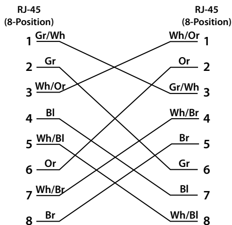
TIA/EIA 568A Crossover CAT5e or CAT6
