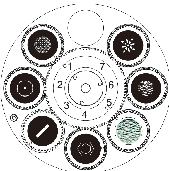
Drehendes Goborad
