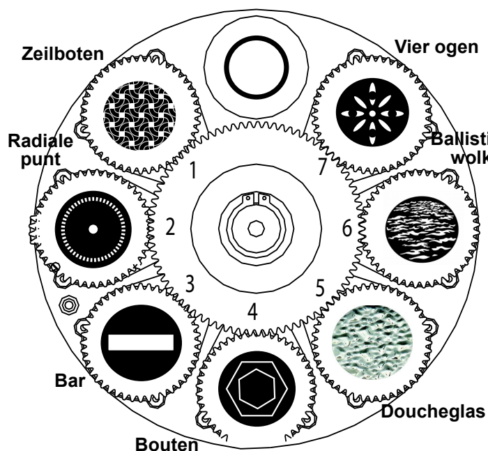
Roterend gobowiel
