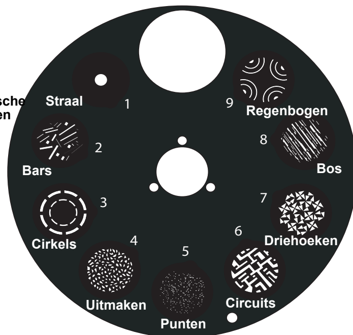
Statisch gobowiel
