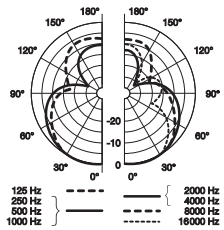
Diagrama polar (hipercardióide)
