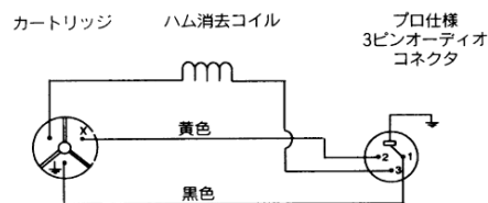
内部接続図
