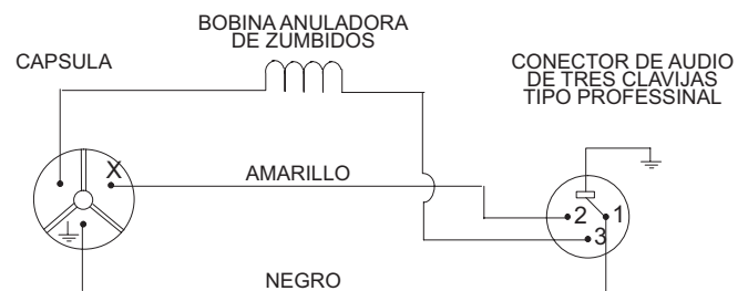
CONEXIONES INTERNAS
