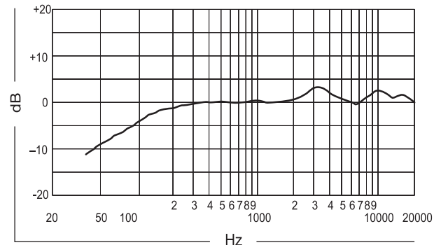
RESPUESTA DE FRECUENCIA TÍPICA
