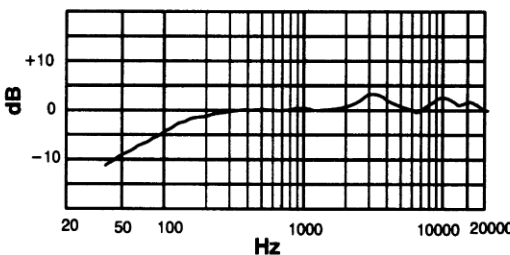
典型频率响应 图 1
