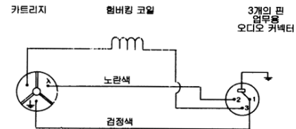
내부 연결도 그림 2
