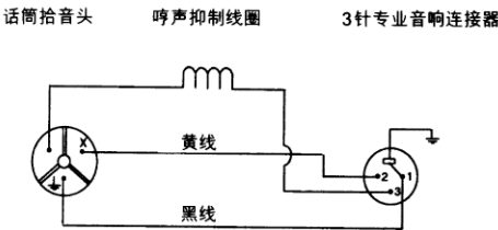
内部连接 图 2
