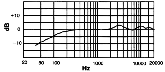
일반적인 주파수 응답 그림 1
