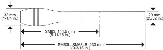
DIMENSIONES GENERALES
